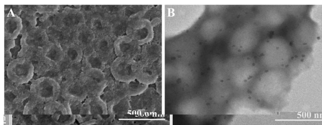
Fig. 5 SEM and TEM images of SF nanocapsules.
